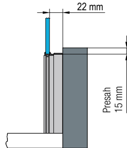
Detail A – pohľad spredu
