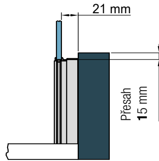
Detail A - pohľad spredu
